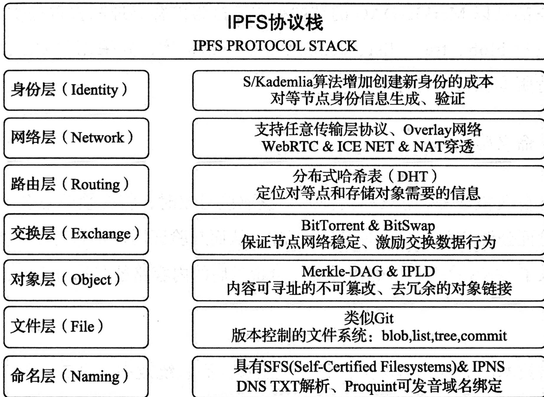
图 1-6 IPFS 协议栈
